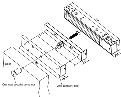
FEM3500 & FEM3500M
